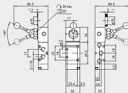
90°- HEBEL 5/2 1/8"
