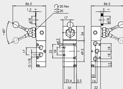
90°- HEBEL 5/2 1/8"
